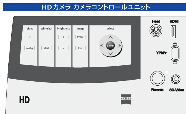
操作パネル及び接続端子概観図
