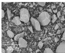
高清掃シリカSEM像(×3000)
