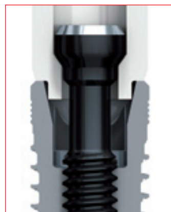
ノーベルプロセラ インプラント ブリッジ用 ショルダー・シーティング
